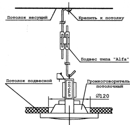
Рис. 1. Крепление громкоговорителя
